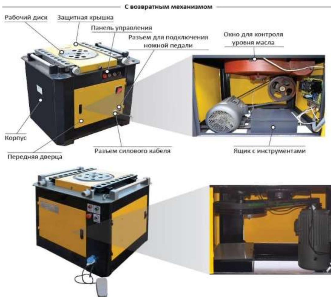
Рис. 1 - Общий вид GW40A, GW50A
